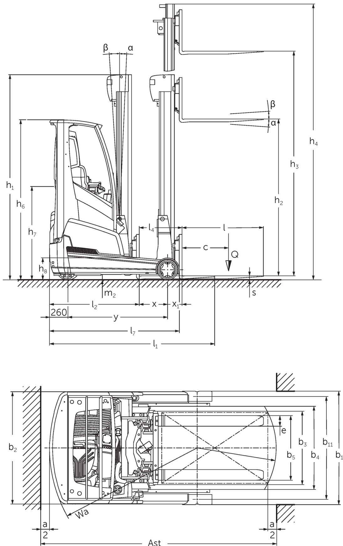
Dibujo técnico, ficha técnica ETV 216i
